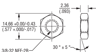
HEX NUT
