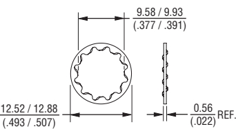
LOCKWASHER
