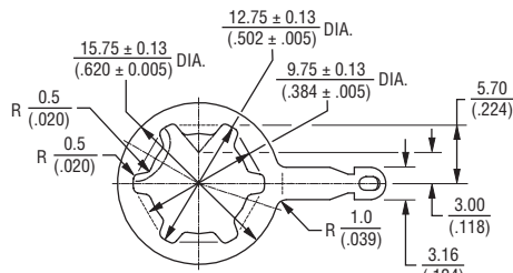
SOLDER LUG WASHER
